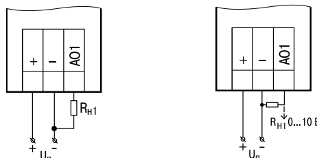
Схема подключения к аналоговому выходу токовой нагрузки
