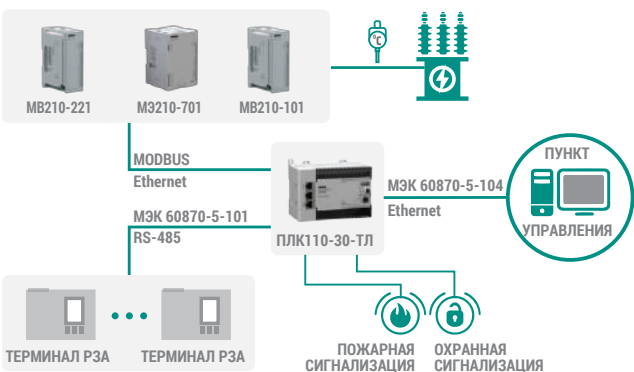
Система телемеханики распределительной трансформаторной подстанции РТП 35/6(10) кВ
