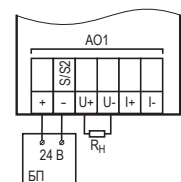
Подключение нагрузки к ВЭ типа У
