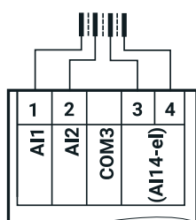
Подключение кондуктометрических датчиков: четырехпроводная схема
