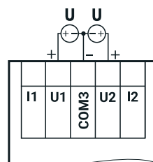
Подключение датчиков с выходом в виде напряжения
