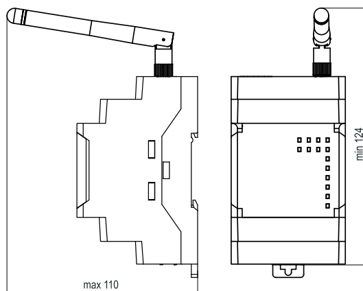
Габаритные размеры Pх210 с антенной
