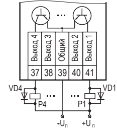
Подключение дискретных выходов типа К ПР200-х.5, ПР200-220.25
