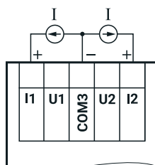
Подключение датчиков с выходом в виде тока
