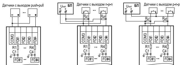
Подключение к входам типа «ДС» датчиков с выходом push-pull
