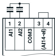
Подключение кондуктометрических датчиков: двухпроводная схема
