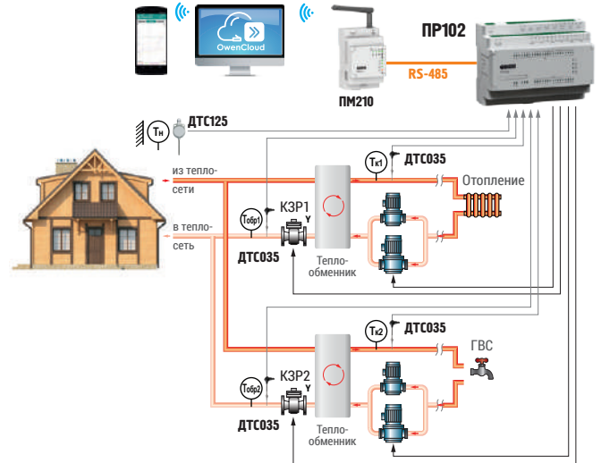
Управление отоплением и ГВС
