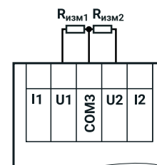
Подключение резистивных датчиков
