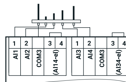
Подключение кондуктометрических датчиков: схема подключения для дискретного режима
