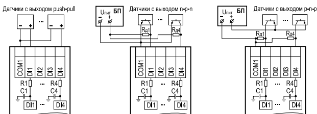
Подключение к входам типа «Д» датчиков с выходом push-pull
