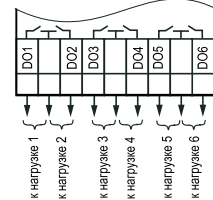
Схема подключения ВЭ типа «Р»
