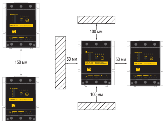
Монтировать приборы вплотную запрещено!
