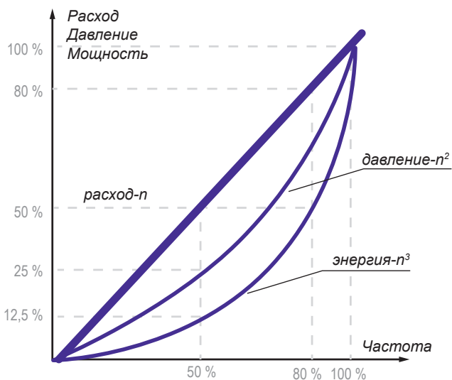
Рис. 1. Зависимость расхода, давления и энергопотребления от числа оборотов
