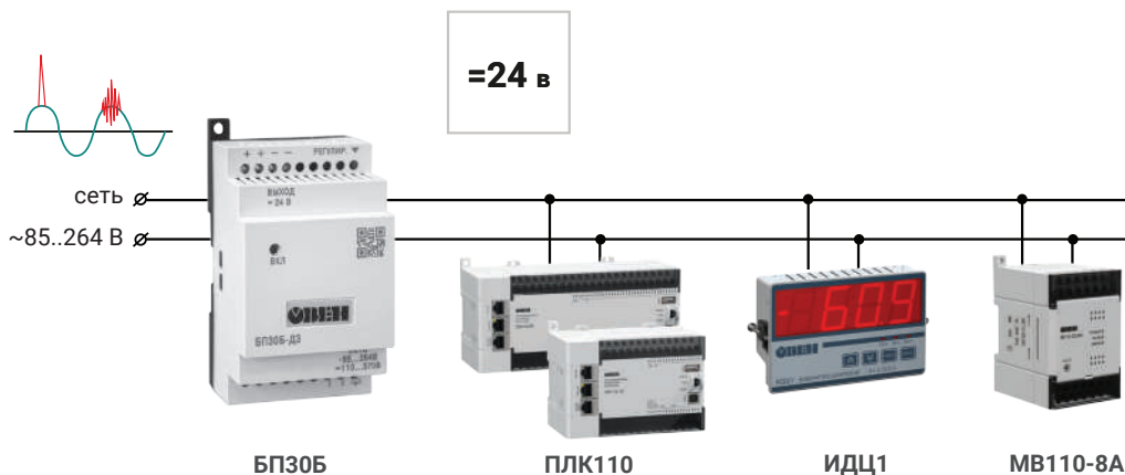
Система контроля и регулирования температуры
