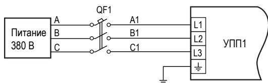
Схема подключения питания УПП1
